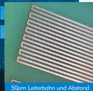
50µm Leiterbahn und Abstand
