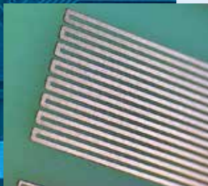
50µm Leiterbahn und Abstand
